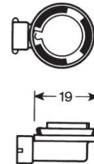
Cód. 80720 116 4 H11, 12V 55W Zócalo: PGJ 19 Uso: alta o baja
