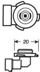
Cód. 80720 116 3 Hb3 9005, 12V 65W Zócalo: P 20d Uso: alta y baja
